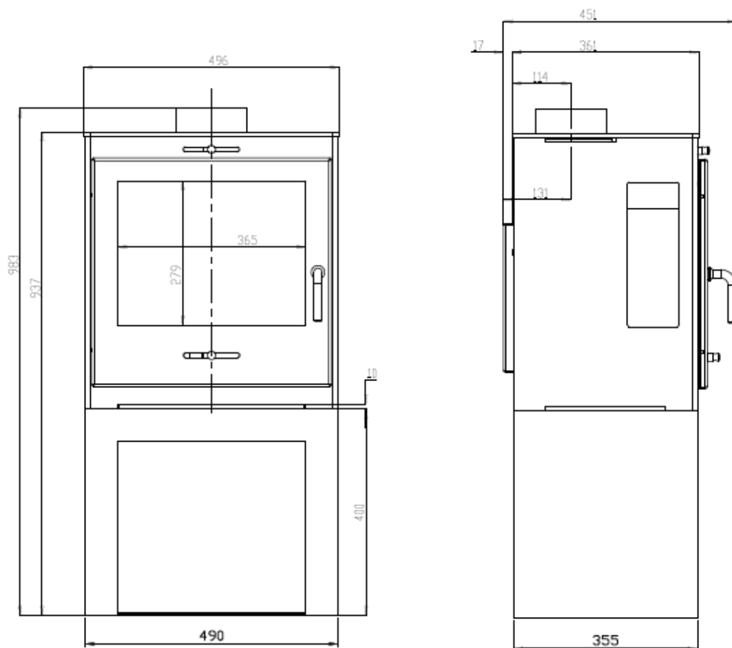
Technický výkres hede 1D:
