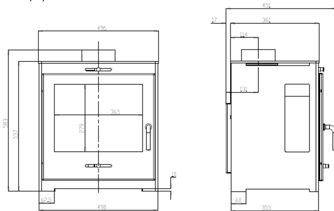
Technický výkres hede 1:
